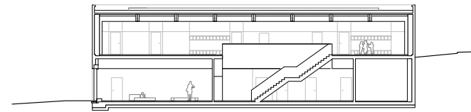
Querschnitt
