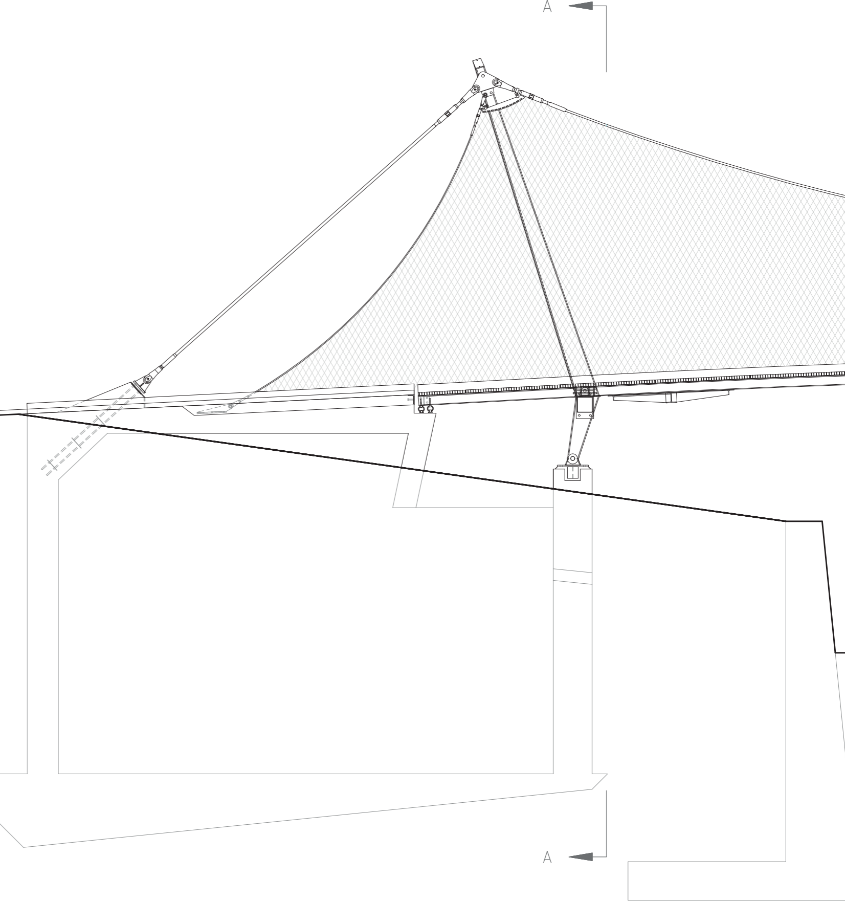
LÄNGSSCHNITT
