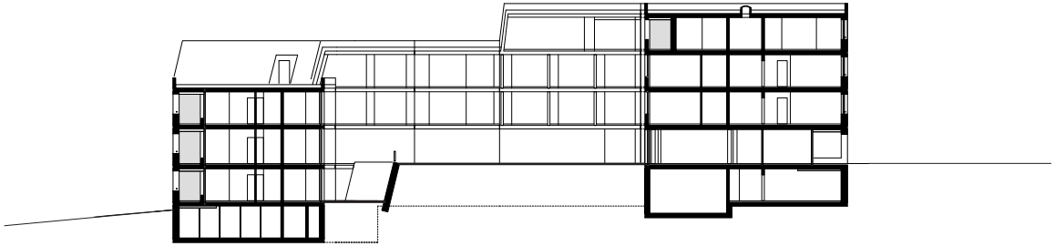
SCHNITT NORD I AA
