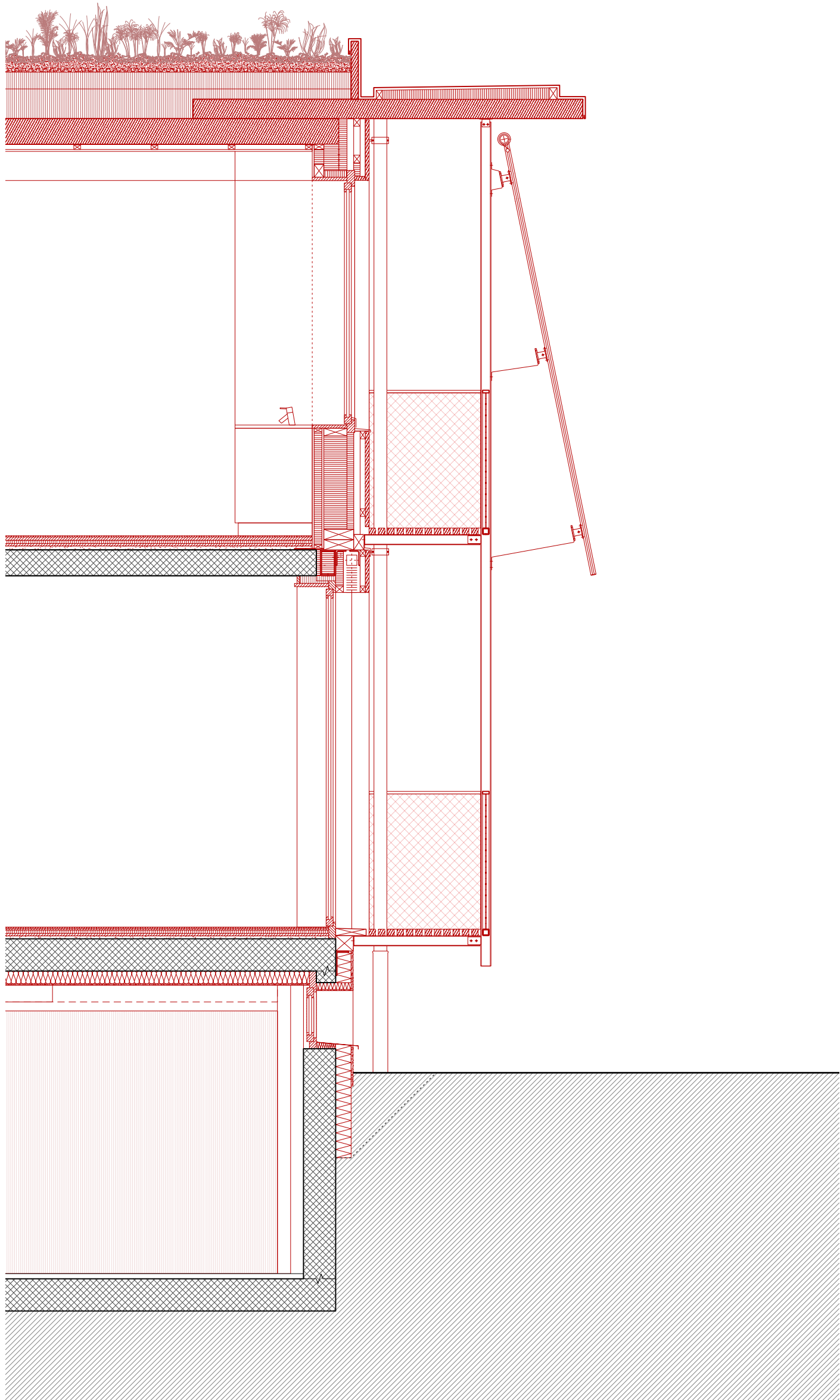
Detailschnitt 1:35
