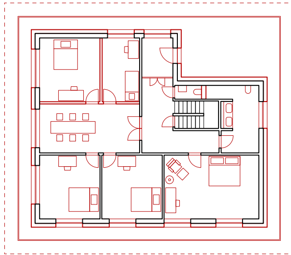
Grundriss Erdgeschoss 1:250
