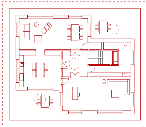
Grundriss Obergeschoss 1:250
