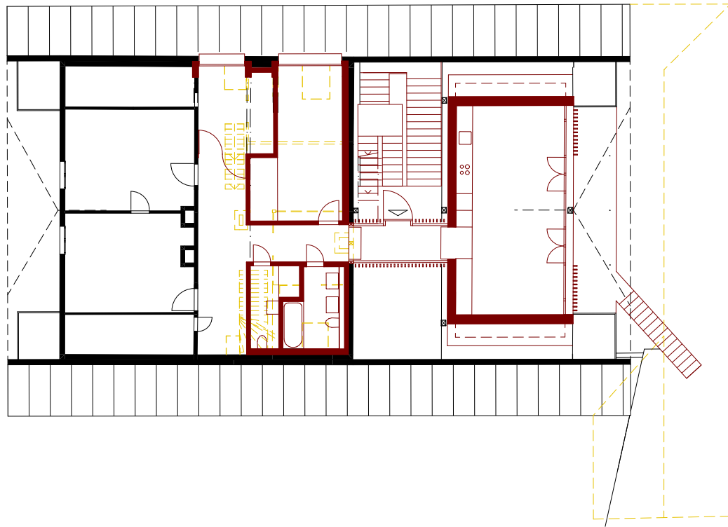
Grundriss Erdgeschoss
