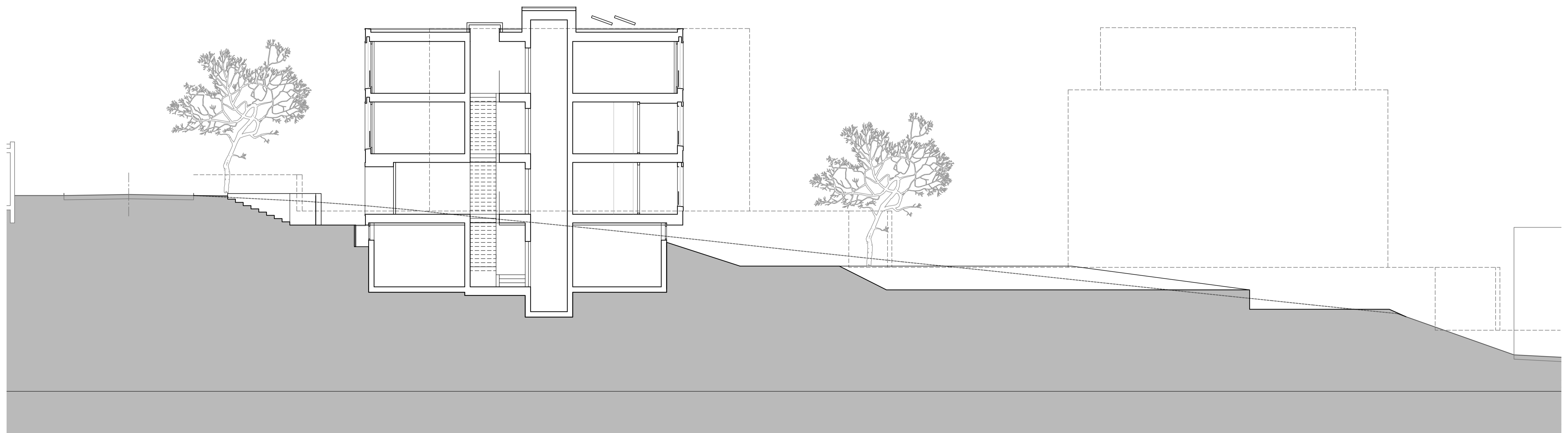
COUPE B_B
